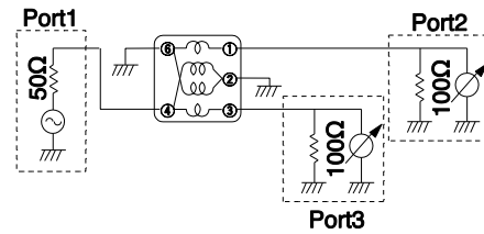
2) #617DB-1674=P3 (Impedance Ratio=50Ω:200Ω)
