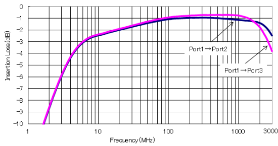
3) #617DB-1675=P3 (Impedance Ratio=50Ω:200Ω)
